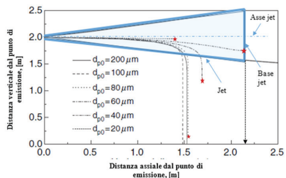
Figura 6. Immagine tratta da Xie et al. (2007). Distanza verticale ed assiale dalla bocca a temperatura dell'aria di 20°C e umidità dell'aria circostante pari a RH = 50%. Le distanze sono state calcolate per velocità di lancio pari a 10 m/s, cioè prossima a quella media di un colpo di tosse (11.7 m/s) e più del doppio di quella tipica durante l'at-
