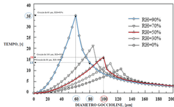
Figura 4. Curva tratta da [2] al variare delle condizioni di umidità relativa (RH) in ambiente. La temperatura ambientale è assunta costante e pari a 18 \text{ }^\circ\text{C} . h
